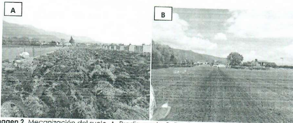
Imagen 2. Mecanización del suelo. A. Predio arado. B. Predio Nivelado
